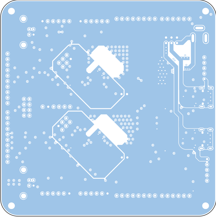
VCC (Scale 1:1)
