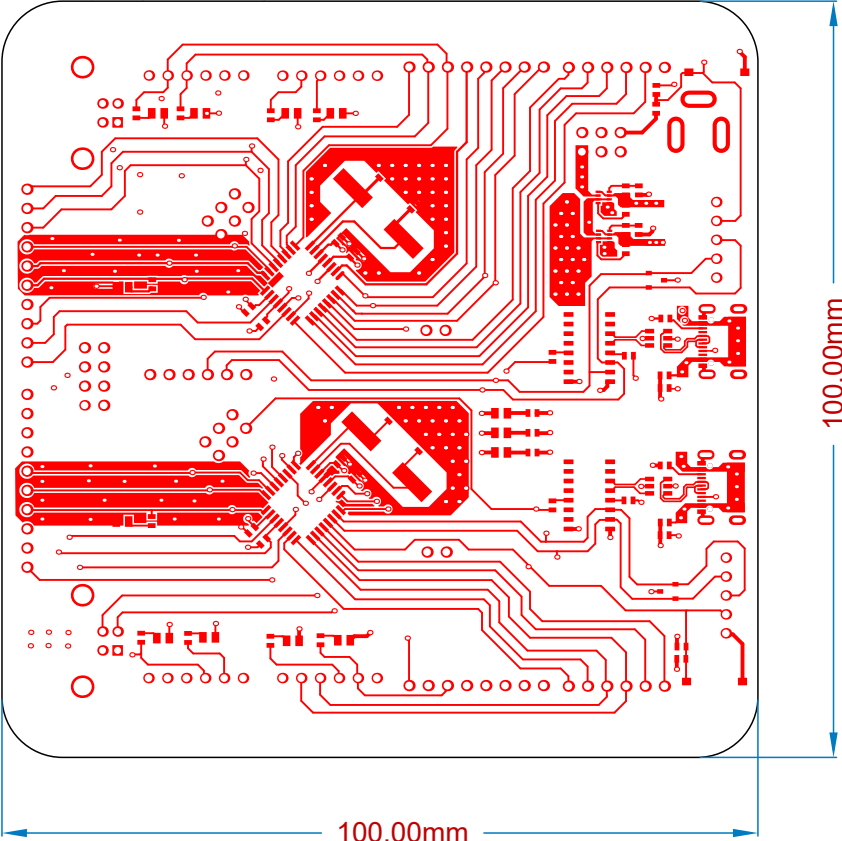
Top Layer (Scale 1:1)
